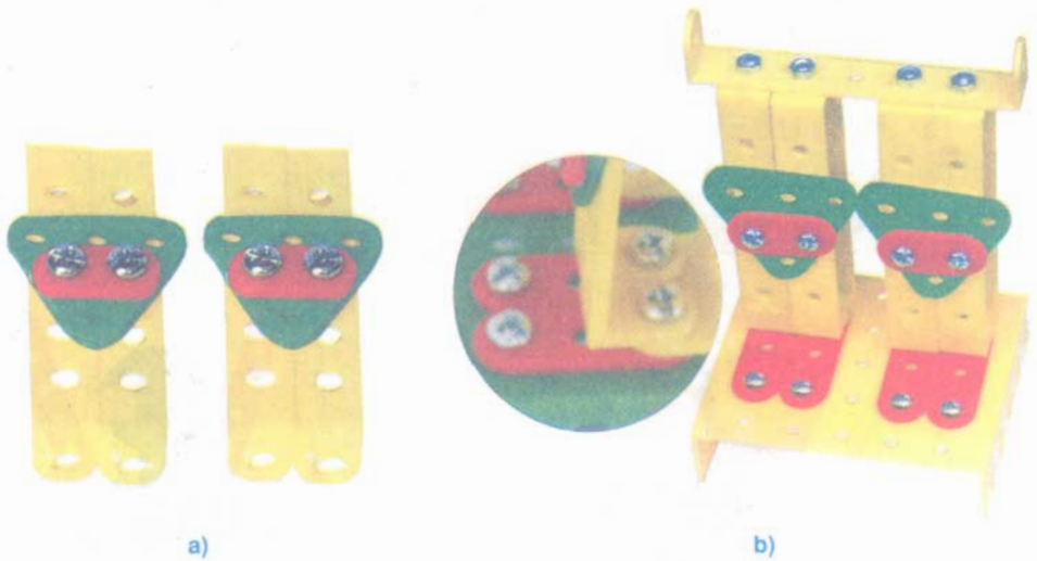
Hình 2. Lắp chân và thanh đỡ thân rô-bốt
